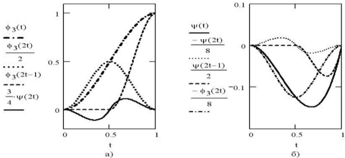
3-сүрөт. Функциялардын графиктери: а) \phi_3(t) , \frac{1}{2}\phi_3(2t) , \phi_3(2t-1) , \frac{3}{4}\psi(2t) ; б) \psi(t) , -\frac{1}{8}\psi(2t) , \frac{1}{2}\psi(2t-1) , (\text{Симметриянын эсебинен ар бир сүрөттүн жарымы гана көрсөтүлгөн}) .
